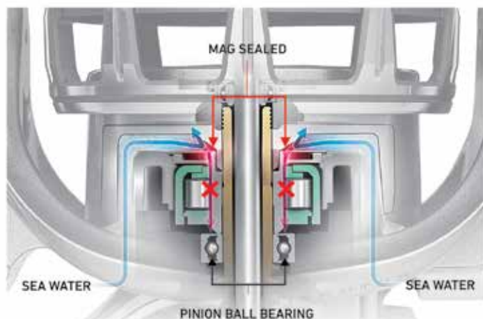
Usporedba rola sa i bez Mag Sealed. Izvor: DAIWA Intern. Service Dept.
